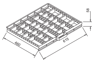
GAVETA PEQUENA Divisórias Removíveis Vãos a partir de 90x25mm
